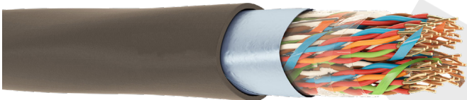
JE-2Y(St)2Y xDSL
