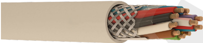
LI2YCY
